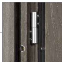
- komplet 3 zawiasów Ø 16 z regulacją 3D - 3 bolce antywyważeniowe - 2 uszczelki
