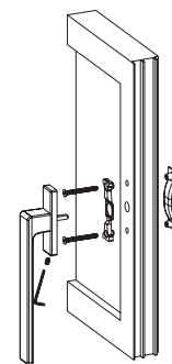
MONTAŻ KLAMKI OKIENNEJ I BALKONOWEJ WINDOW HANDLE ASSEMBLY
