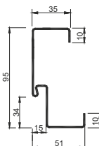
Ościeżnica stalowa 10/54, 10/54 AKU
