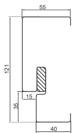
Ościeżnica stalowa T/54, T/54 AKU
