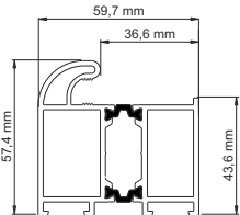
Profil ościeżnicy ALU/54
