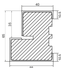
Ościeznica drewniano-stalowa DS/54
