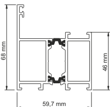
Profil naświetla
