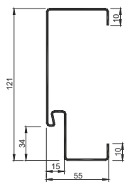
Ościeżnica stalowa S15/54
