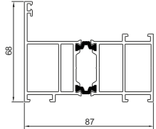
Profil naświetla
