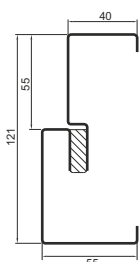
Ościeznica stalowa NT/75
