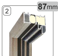
Ościeżnica aluminiowa ALU/90 trzykomorowa z podwójnym uszczelnieniem z przegrodą PCW wypełnioną pianą
