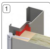
Wypełnienie skrzydła PŁYTA SKALNEJ WEŁNY MINERALNEJ
