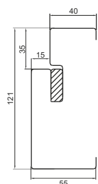
Ościeznica stalowa NT/54
