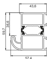
Ościeznica aluminiowa ALU/54
