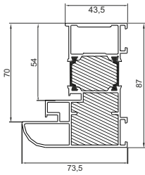
Ościeznica aluminiowa ALU/90
