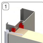
Wypełnienie skrzydła PIANA POLIURETANOWA
