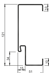
Ościeżnica stalowa 15/54, 15/54 AKU
