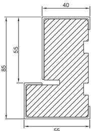
Ościeznica drewniano-stalowa DS/75
