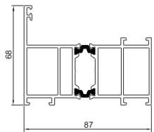
Profil naświetla
