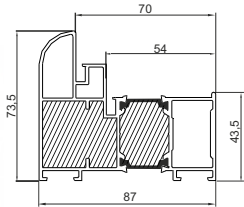
Profil ościeżnicy ALU/90
