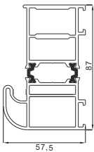
Ościeznica aluminiowa ALU/75
