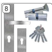
Klamka SIGMA inox, wkładka+wkładko-gałka system jednego klucza standard
