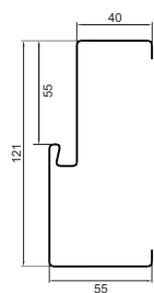
Ościeznica stalowa S15/75
