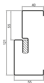
Ościeznica stalowa T/75
