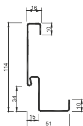
Ościeżnica stalowa 11/54, 11/54 AKU
