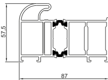
Profil ościeżnicy ALU/75
