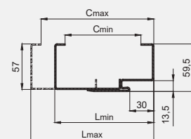
Profil ościeżnicy stalowej regulowanej z kątownikiem domykającym T57
