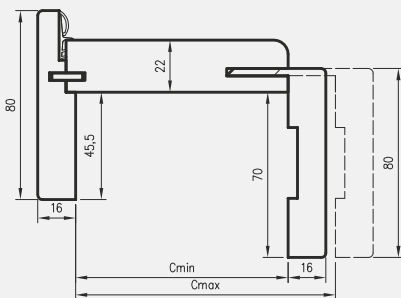
Profil ościeżnicy
