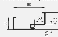
Profil ościeżnicy stalowej
