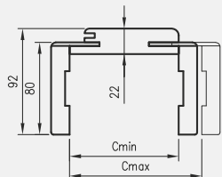
Przekrój OR/ORC z ką. T63
