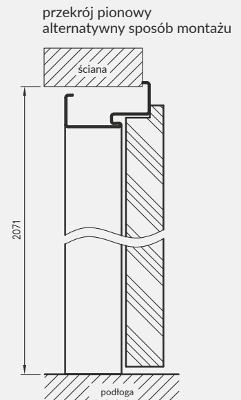
przekrój pionowy ościeżnicy stalowej stałej
