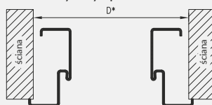
Przekrój poprzeczny alternatywny sposób montażu
