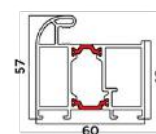
Rysunek techniczny
