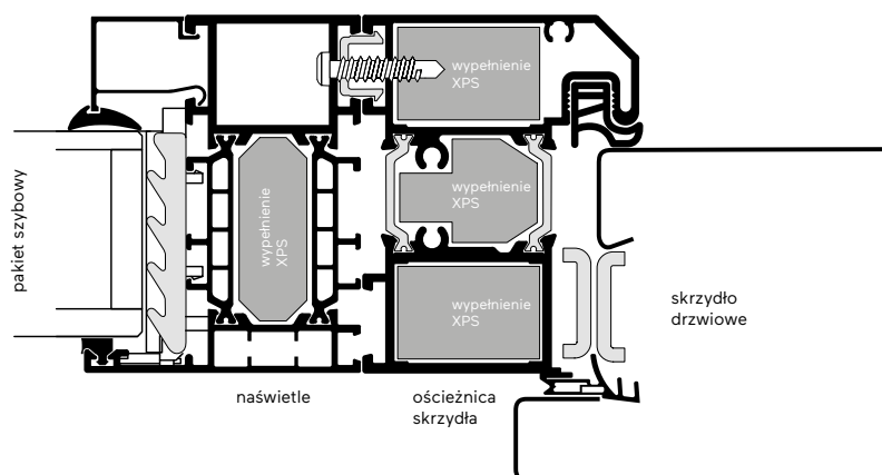
Złożenie drzwi Comfort 73 z naświetłem bocznym
